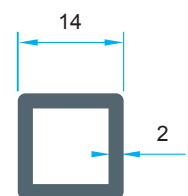
Code: P-1336 0,257 kg/m
